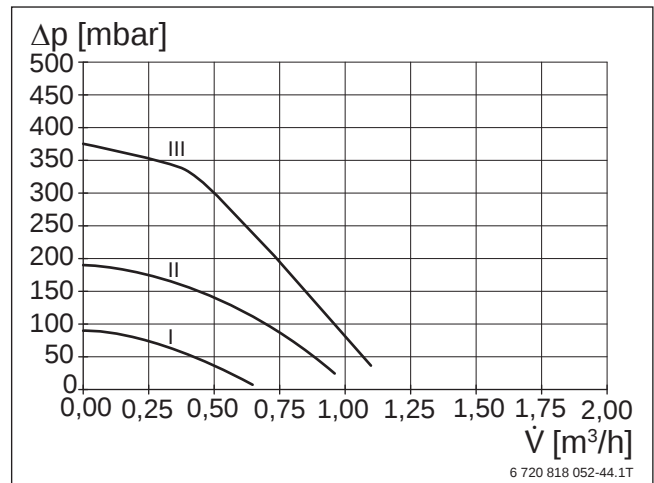
Bild 42 Konstante Regelung HSM15
