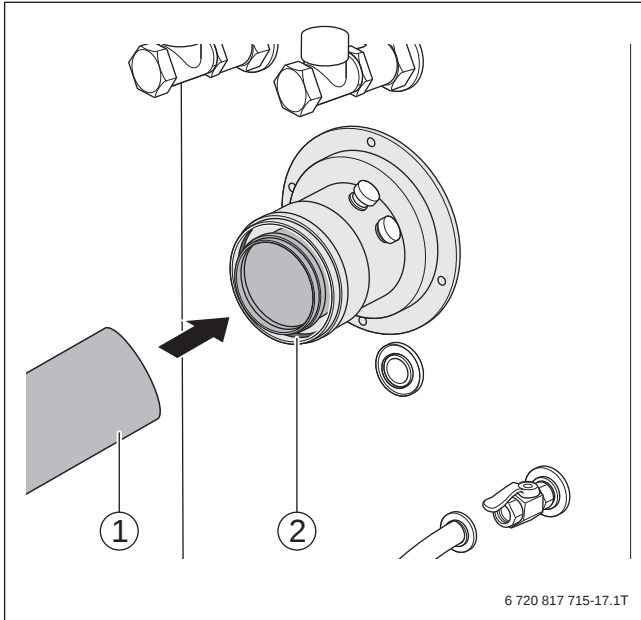
Bild 67 Montage Abgasrohr
