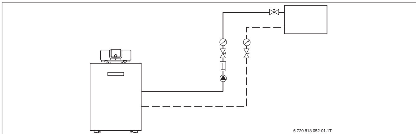
Bild 15 Installationshinweise GC7000F 15 ... 50
