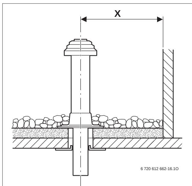
Bild 69 Dachdurchführung Flachdach
