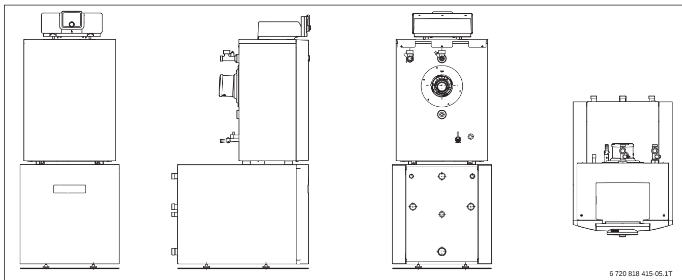
Bild 35 GC7000F 15 ... 50 mit Warmwasserspeicher Stora WST ...-2 HRC
