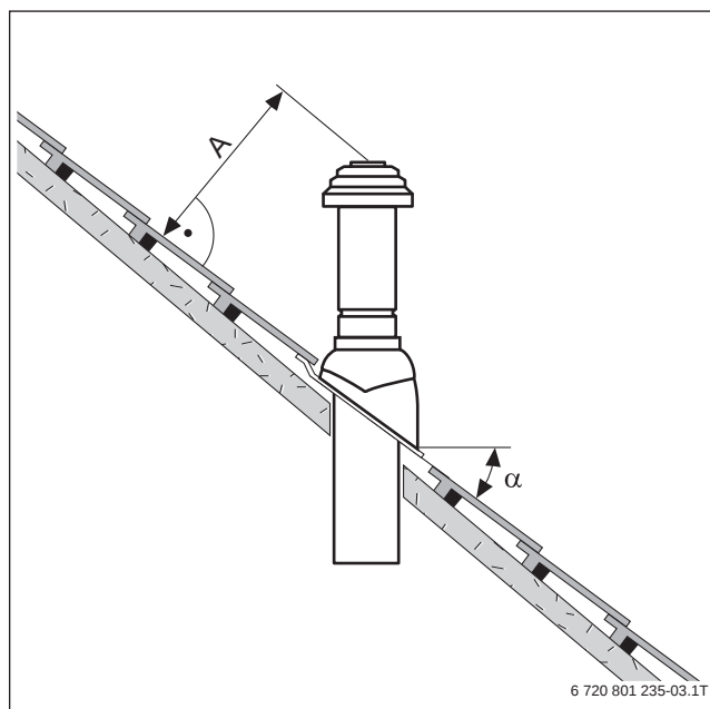
Bild 70 Dachdurchführung Schrägdach
