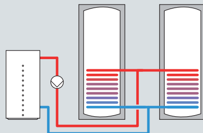
2 Speicher parallel geschaltet
