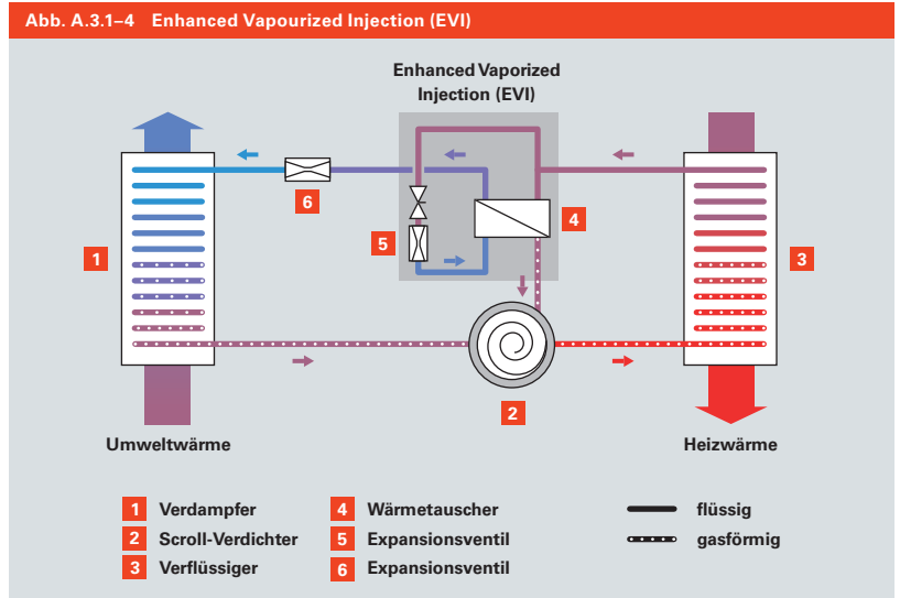
Ein Teil des Kältemittels wird nach der Verflüssigung (3) genutzt, um mithilfe eines zusätzlichen Wärmetauschers (4) und eines weiteren Expansionsventils (5) Dampf zu erzeugen, der wiederum direkt in den Verdichter (2) eingespritzt wird. Das geschieht an dem Punkt, an dem die Verdichtung zu etwa zwei Dritteln abgeschlossen ist. Durch diese Dampfwischeneinspritzung wird der bis hierher verdichtete Kältemitteldampf gekühlt.
