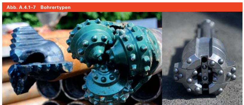
Je nach Untergrund und Sondenmaß werden unterschiedliche Bohrertypen verwendet.
