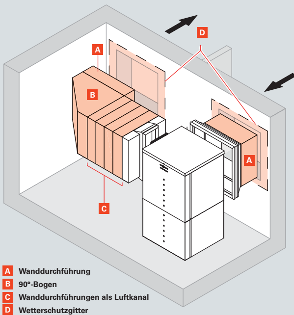
Abb. C.3.4-1 Luftführung bei Innenaufstellung
