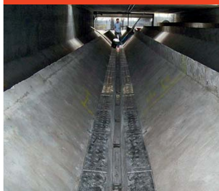
Abb. A.4.5-2 Abwasser-Wärmetauscher
