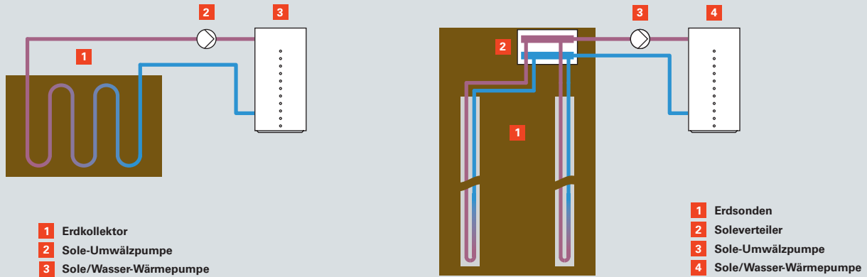
Abb. C.1.1-1 Erdkollektor und Erdsonde
