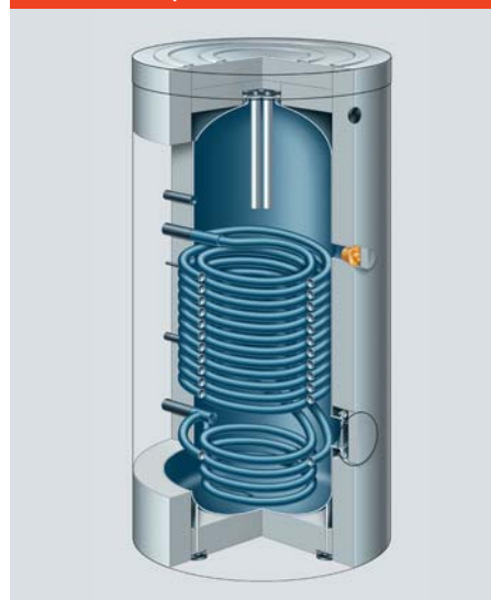
Abb. D.2.1-11 Speicher-Wasserwärmer
