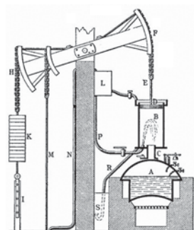
Abb. A.1-1 Dampfmaschine von Newcomen
