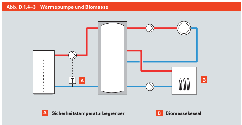
Einbindung eines Biomassekessels in das Wärmepumpensystem.
