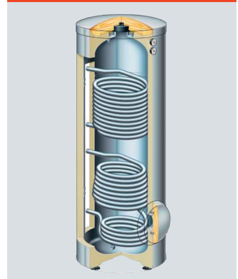
Abb. D.2.1-12 Bivalenter Speicher-Wasserwärmer
