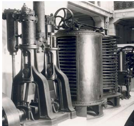
Abb. A.1-3 Linde Kältemaschine von 1877
