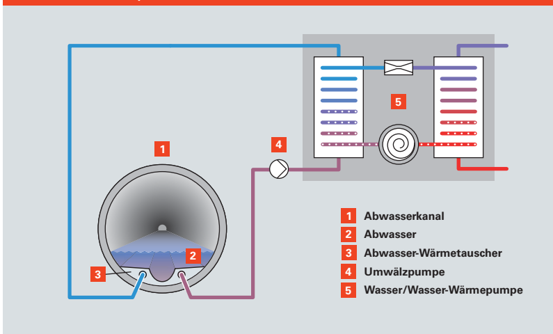
Abb. A.4.5-1 Wärmequelle Abwasser
