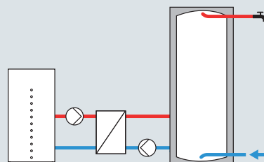
Ladespeicher mit externem Wärmetauscher
