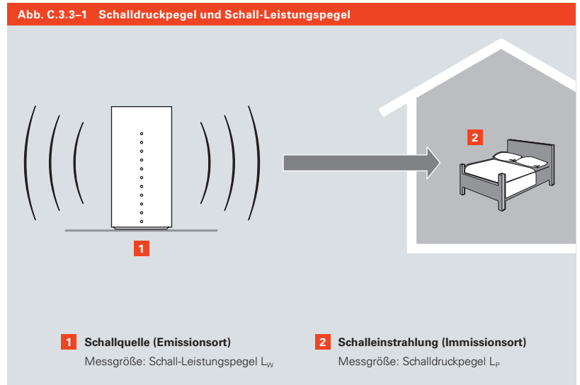
Die Schall-Leistung geht von der Schallquelle aus. Der Schalldruck wird am Ohr empfunden.
