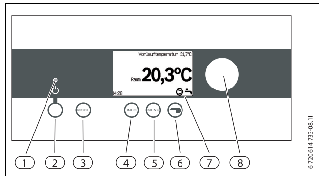
Bild 2 Bedienfeld
